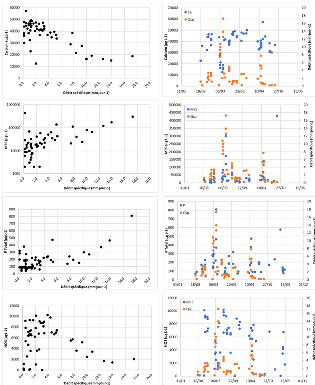
Figure 11. Distribution des concentrations observées en calcium (Ca), matières en suspension (MES), phosphore total (P total) et nitrates (NO 3 ) en fonction du débit spécifique (Qsp) et de la date d'échantillonnage à la station hydrométrique du Grand Marais.
