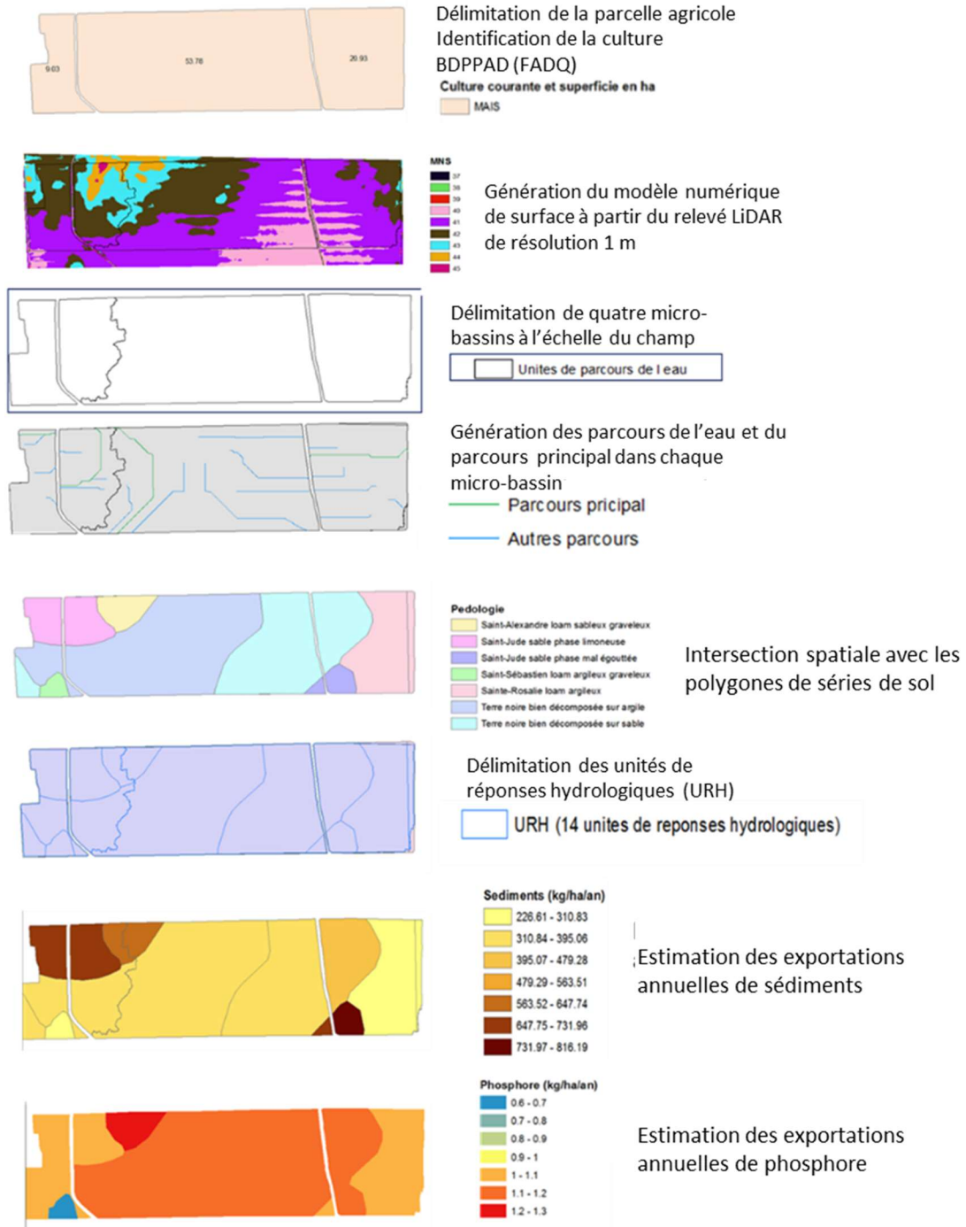
Figure 18. Illustration des différentes étapes de traitement des données à référence spatiale dans GÉODEP pour une portion de territoire à vocation agricole.
