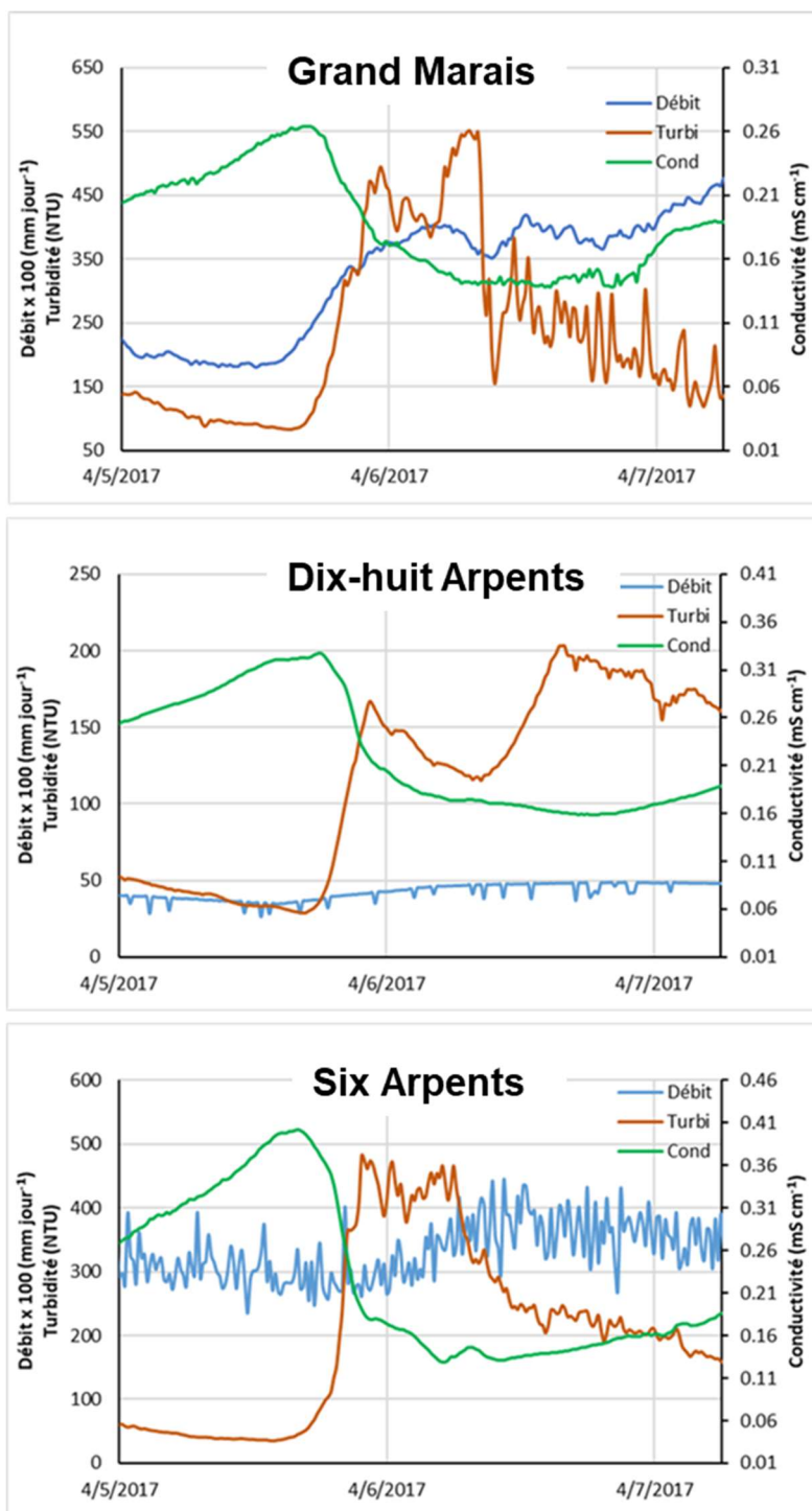
Figure 9. Variation du débit, de la turbidité et de la conductivité au pas de temps de 15 minutes pour la crue du 5 au 7 avril 2017 observée aux trois stations hydrométriques.
