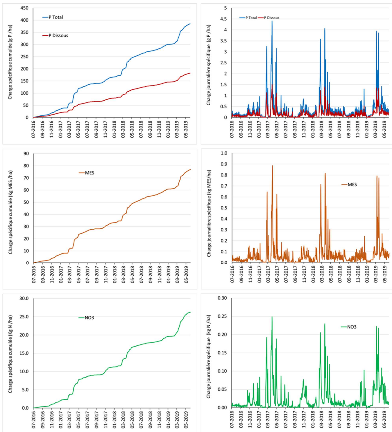
Figure 15. Distribution des flux et charges cumulées de matières en suspension, de phosphore total et dissous, et des nitrates à la station hydrométrique du ruisseau Dix-huit Arpents.
